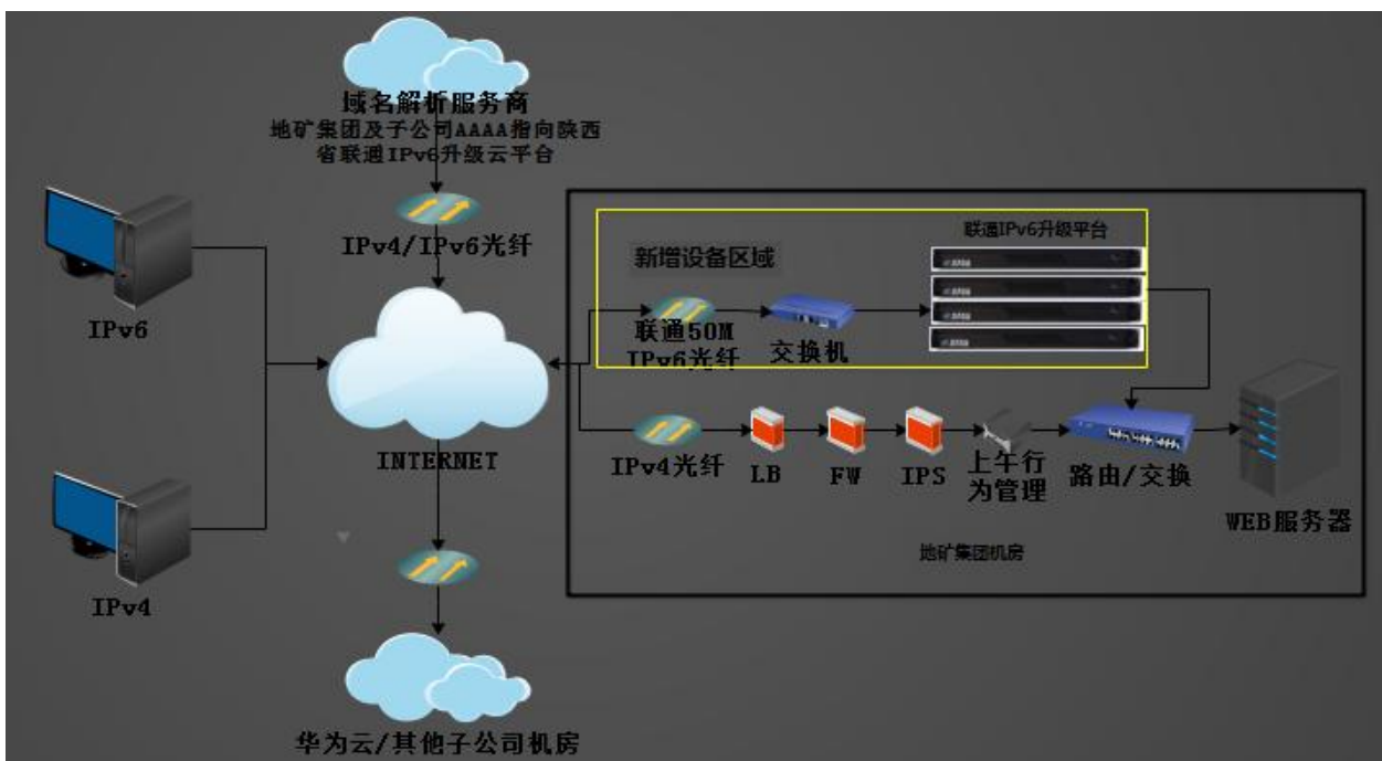
图 1 网站 IPv6 升级网络拓扑
