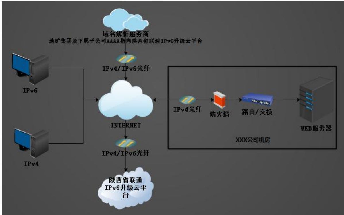
图 2 网站 IPv6 升级网络拓扑
